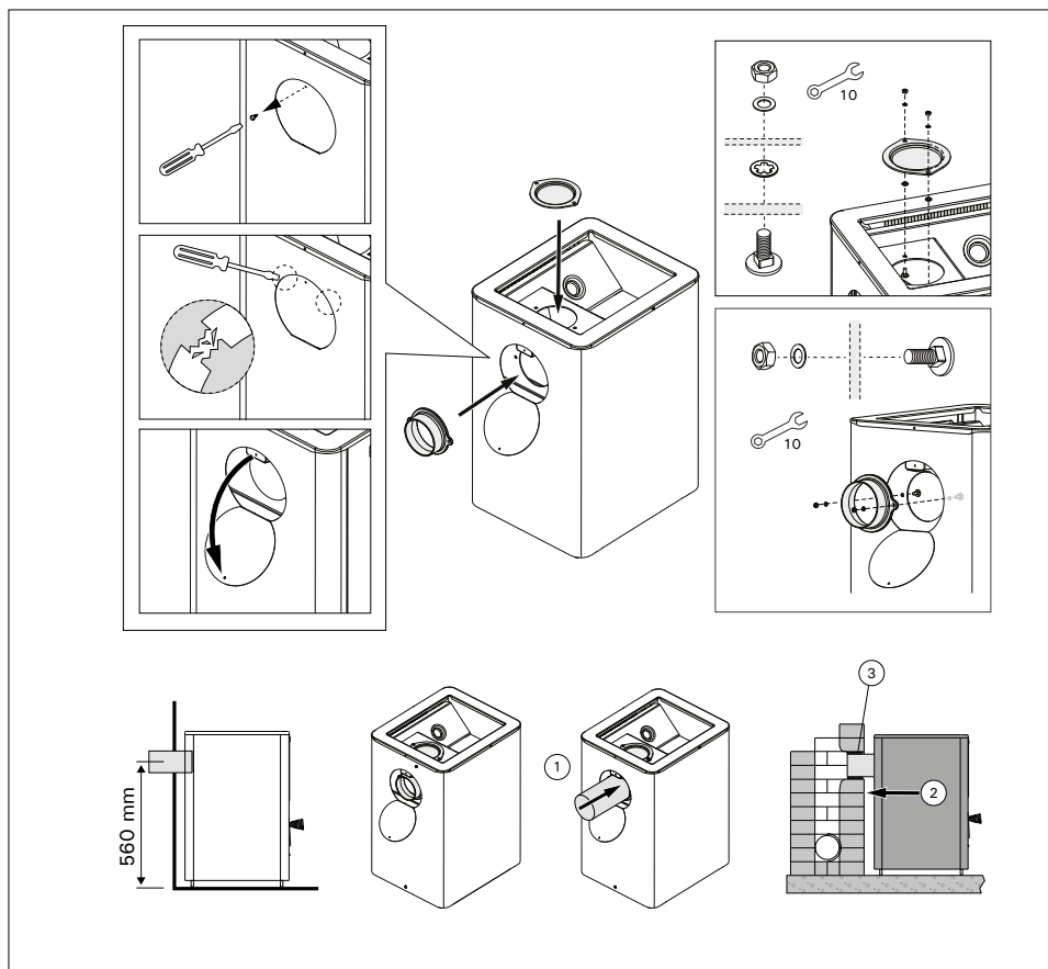
Figuur 11. De kachel aansluiten op een gemetseld rookkanaal via de aansluitopening achter.
