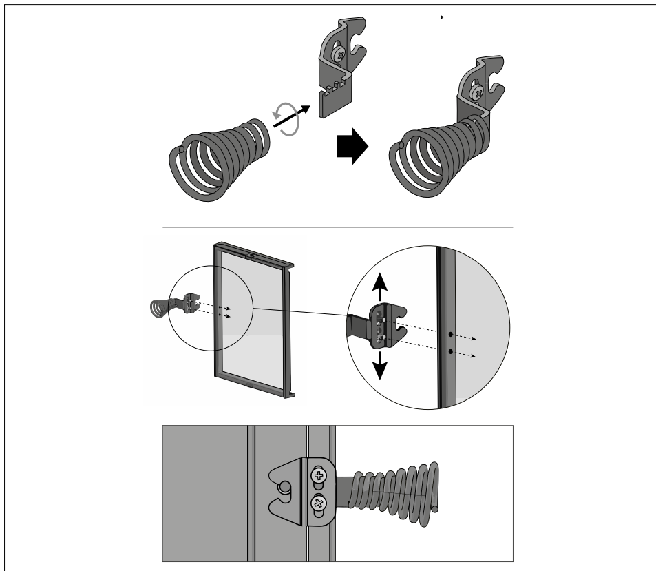
Figure 14. Montage de la poignée.
