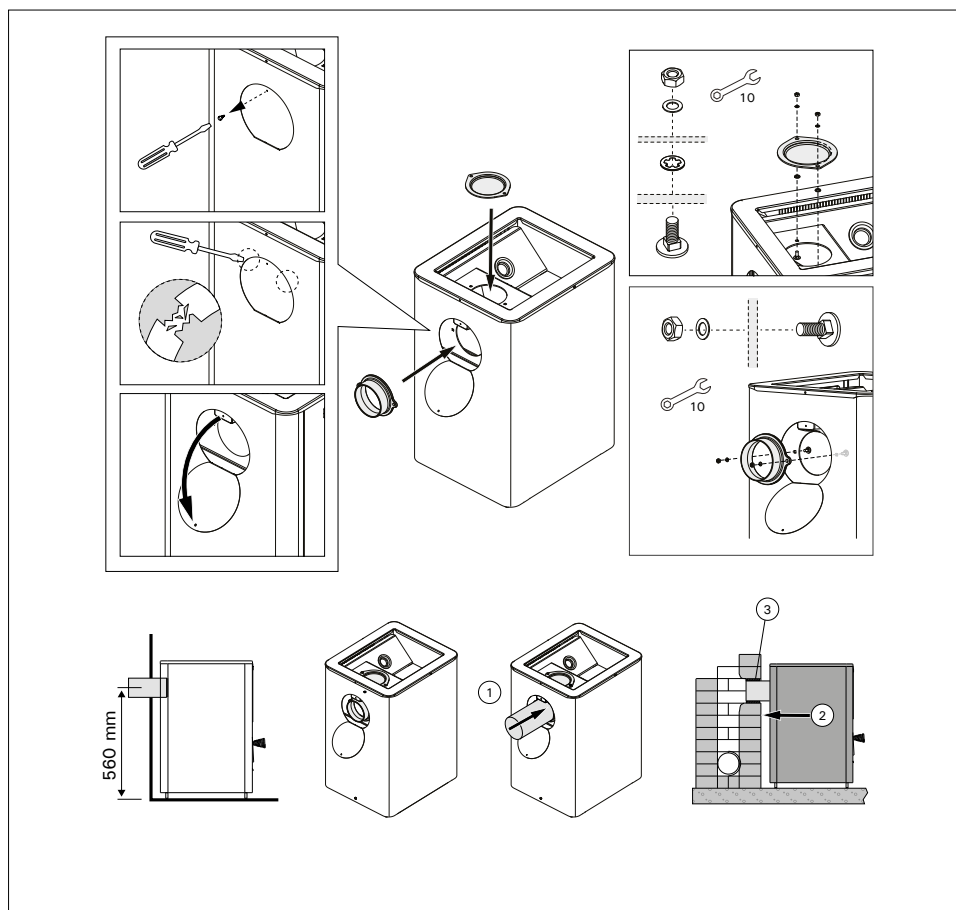
Figure 11. Raccordement du poêle à un conduit maçonné via l'ouverture de raccordement arrière.
