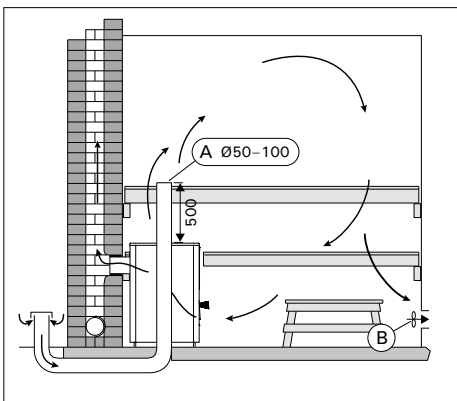
Figure 7. Ventilation mécanique.
