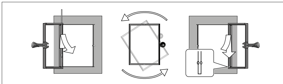
Figure 15. Modification du sens d'ouverture de la porte du foyer.
