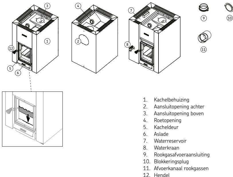
Figuur 1. Onderdelen van de kachel.
