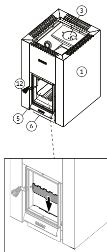
Figure 1. Composants du poêle. Figura 1. Parti della stufa.
