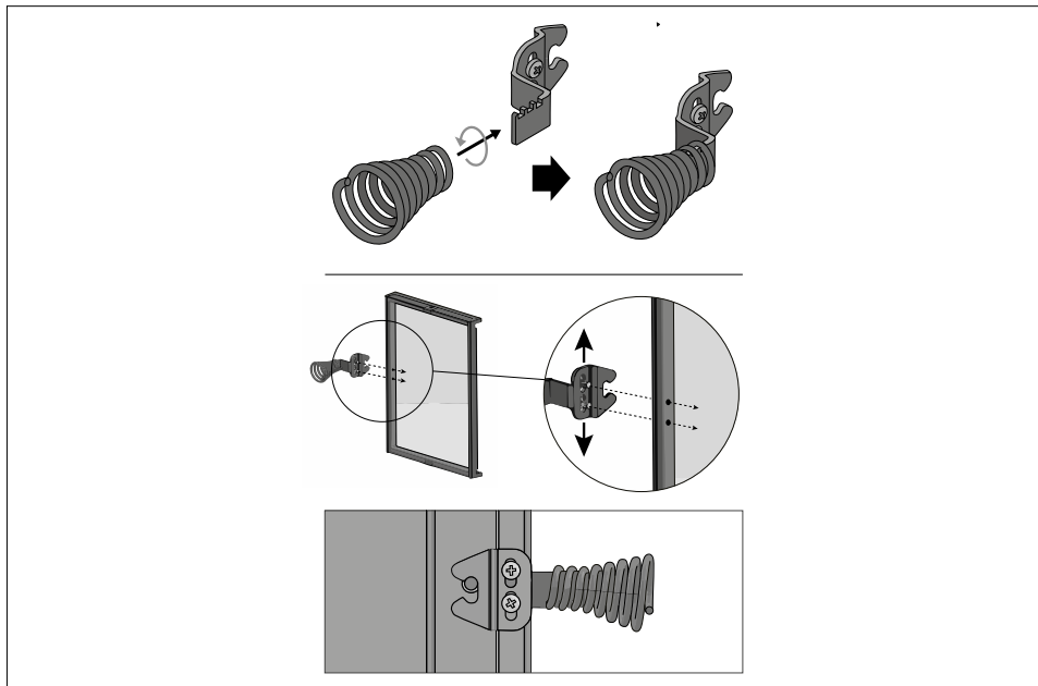
Figuur 14. De handgreep monteren.
