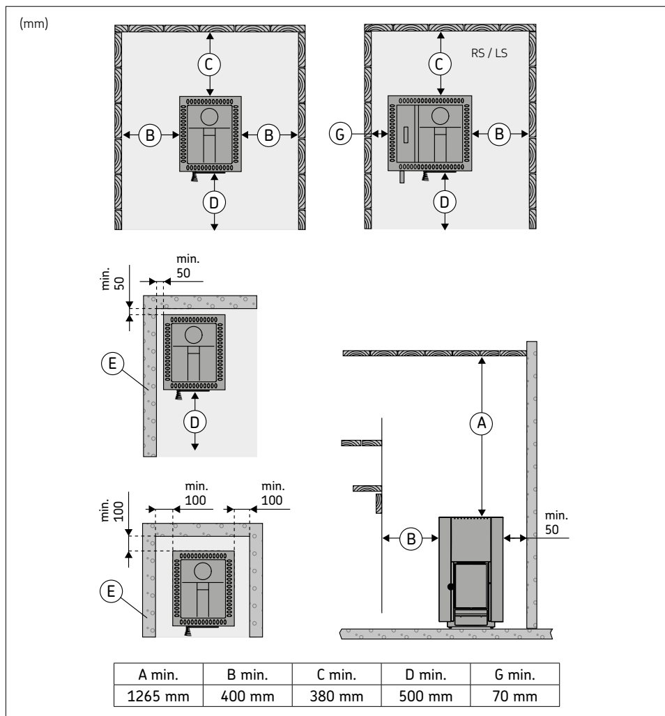
Figure 9. Distances de sécurité.
